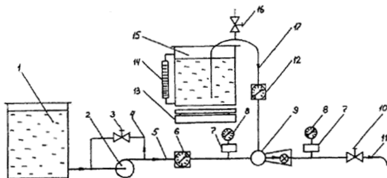
Рис. 2. Установка для определения расхода воды и пенообразователя через дозатор:
